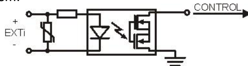
Rys. 18. Schemat elektryczny wejścia EXTi.
