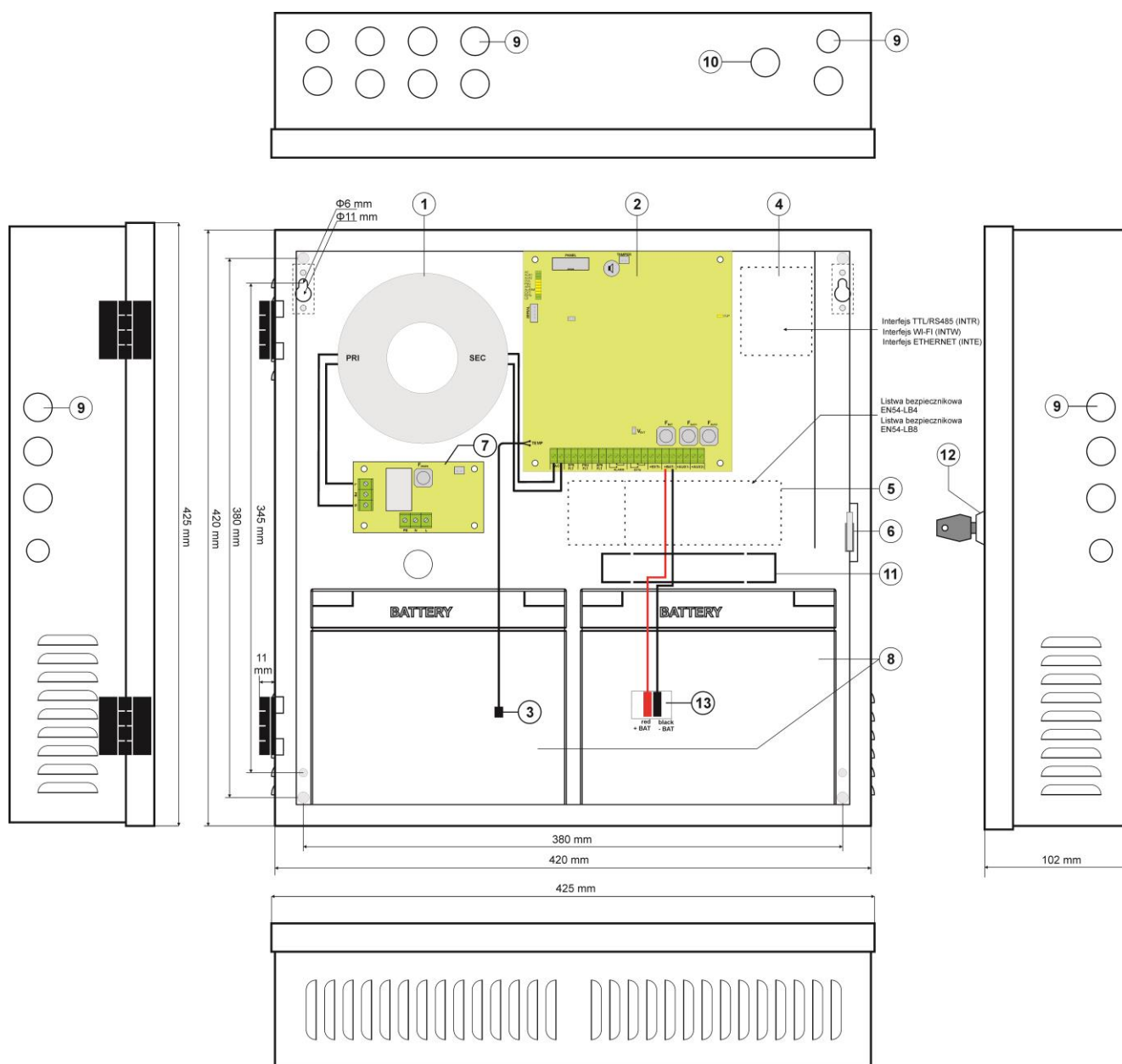
Rys.4. Widok zasilacza.
