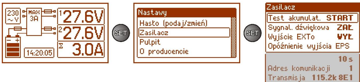
Rys. 25. Ekran „Zasilacz”.
