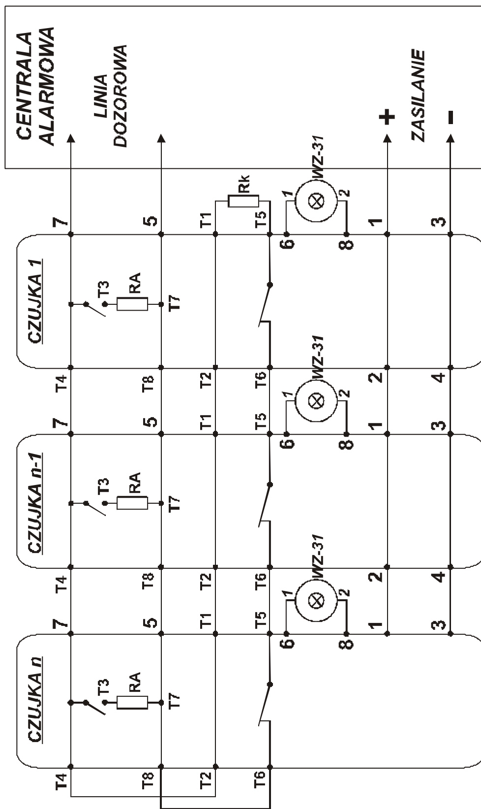
Rys 7. łączenie czujek DOP-6001R w linii dozorowej
